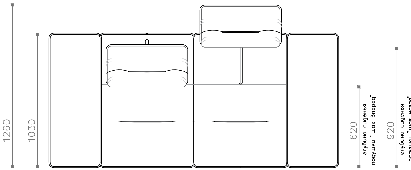
Вид сверху Диван для отдыха 146 с 2мя боковинами (Б+Д 146+Б-224)
