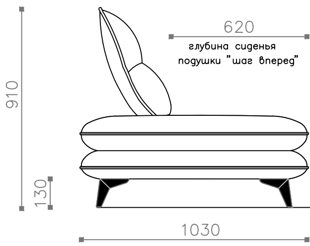
Вид сбоку Диван для отдыха, подушки "шаг вперед"
