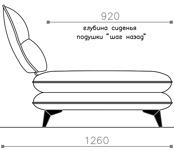
Вид сбоку Диван для отдыха, подушки "шаг назад"
