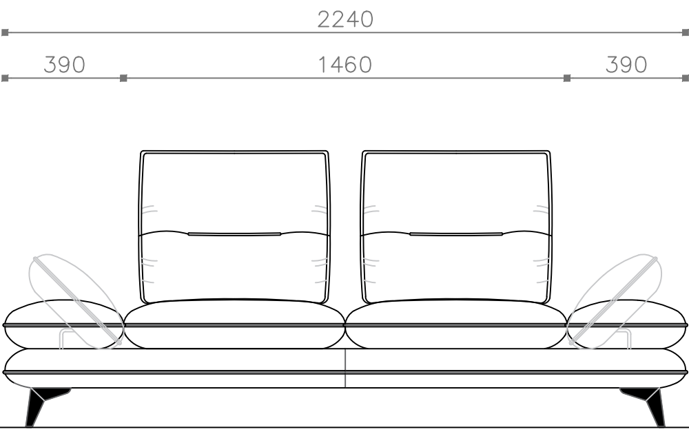
Фронтальный вид Диван для отдыха 146 с 2мя боковинами (Б+Д 146+Б-224)
