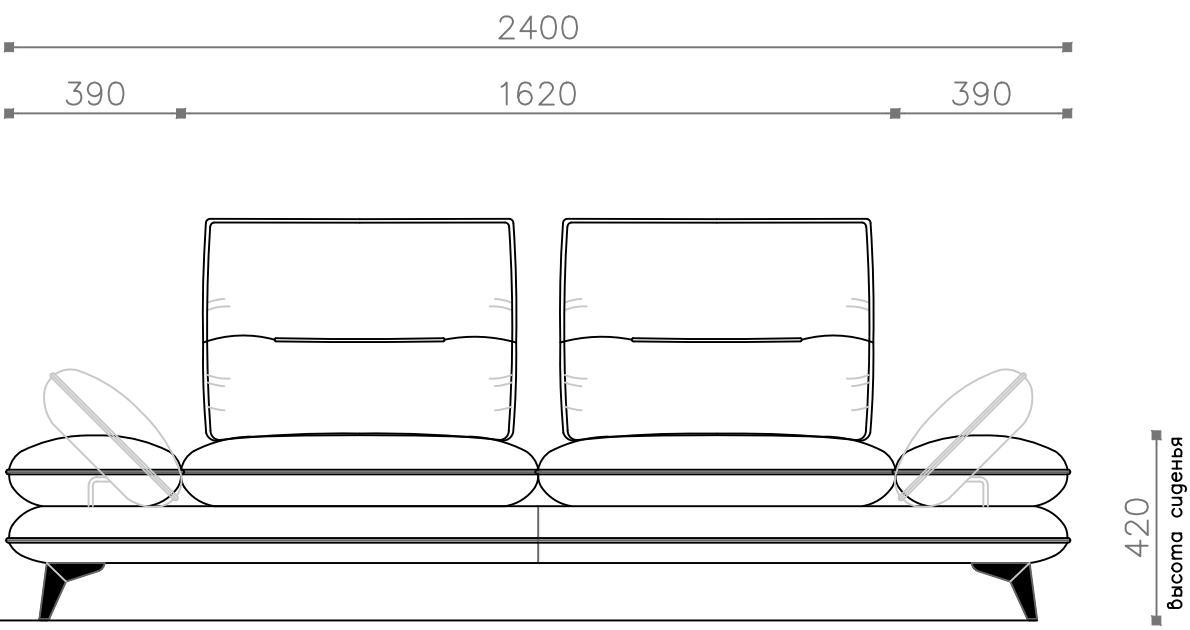
Фронтальный вид Диван для отдыха 162 с 2мя боковинами (Б+Д 162+Б-240)
