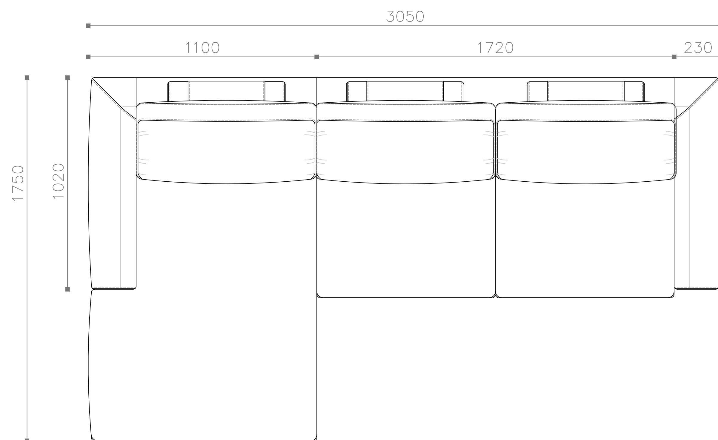
Вид сверху 0мм 110+ДКР 172+Б
