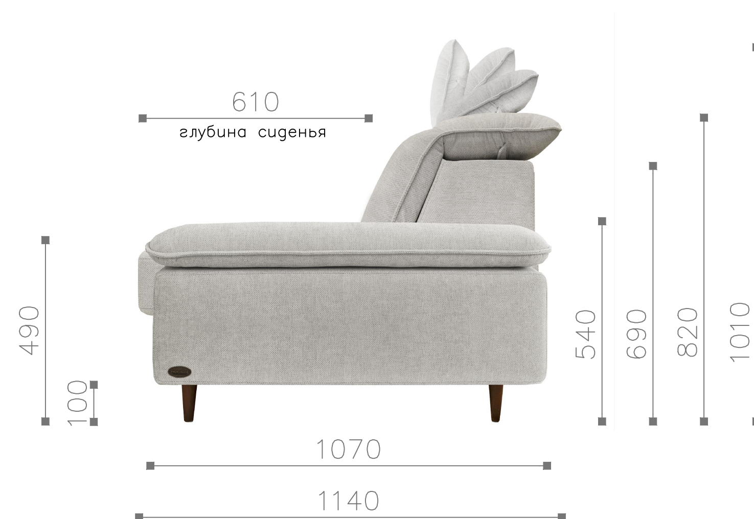
Вид сбоку с боковиной 1 (Б1)
