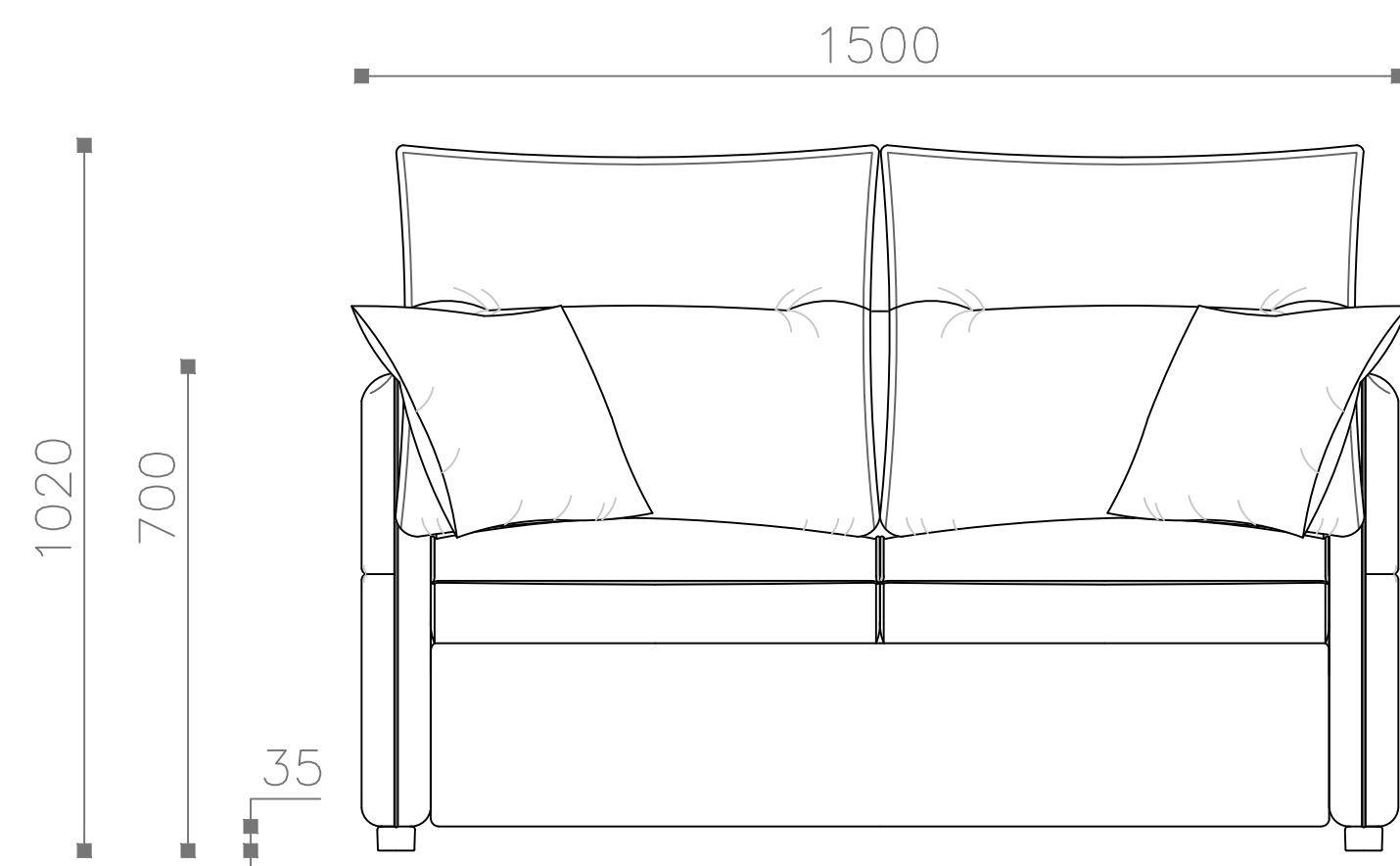
Диван-кровать 150 (ДКР 150) Фронтальный вид
