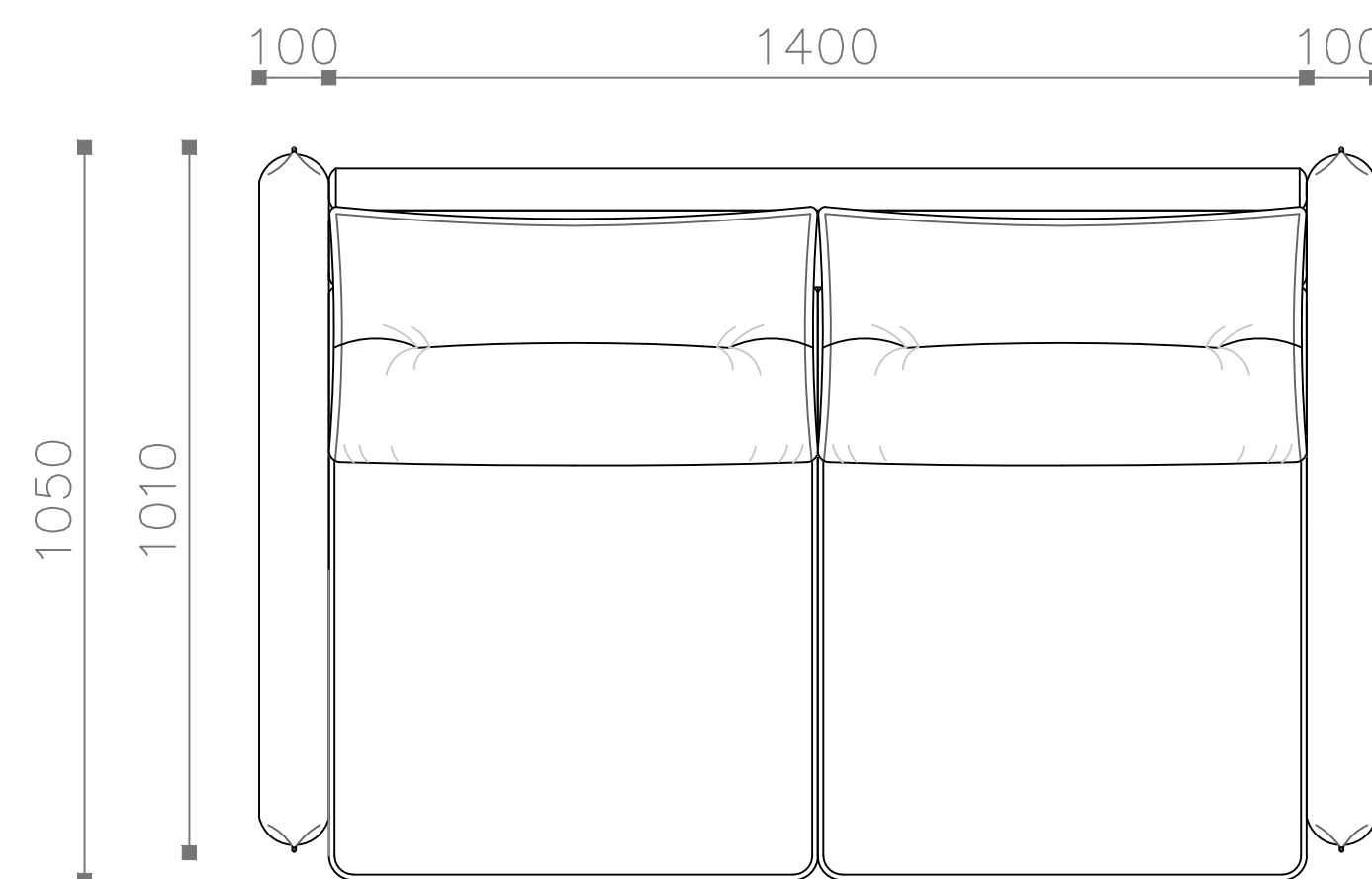
Диван-кровать 160 (ДКР 160) Вид сверху
