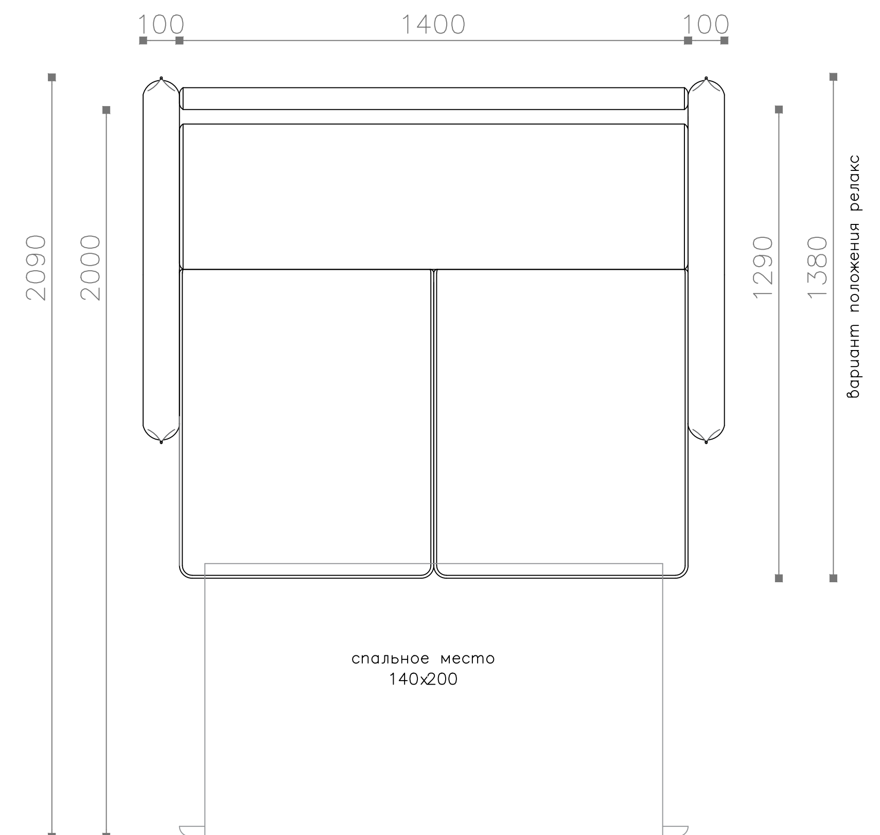
Диван-кровать 160 (ДКР 160) в разложенном виде Вид сверху
