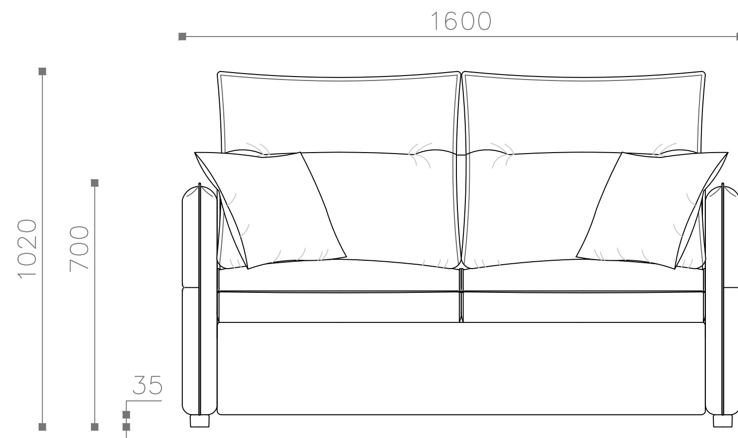
Диван-кровать 160 (ДКР 160) Фронтальный вид
