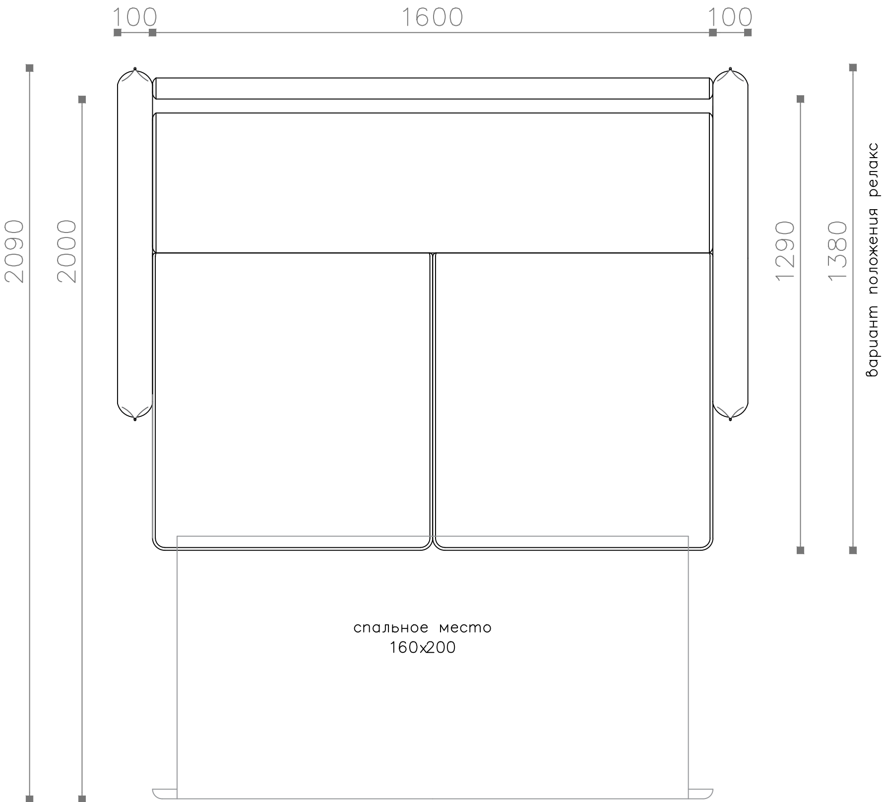
Диван-кровать 180 (ДКР 180) в разложенном виде Вид сверху
