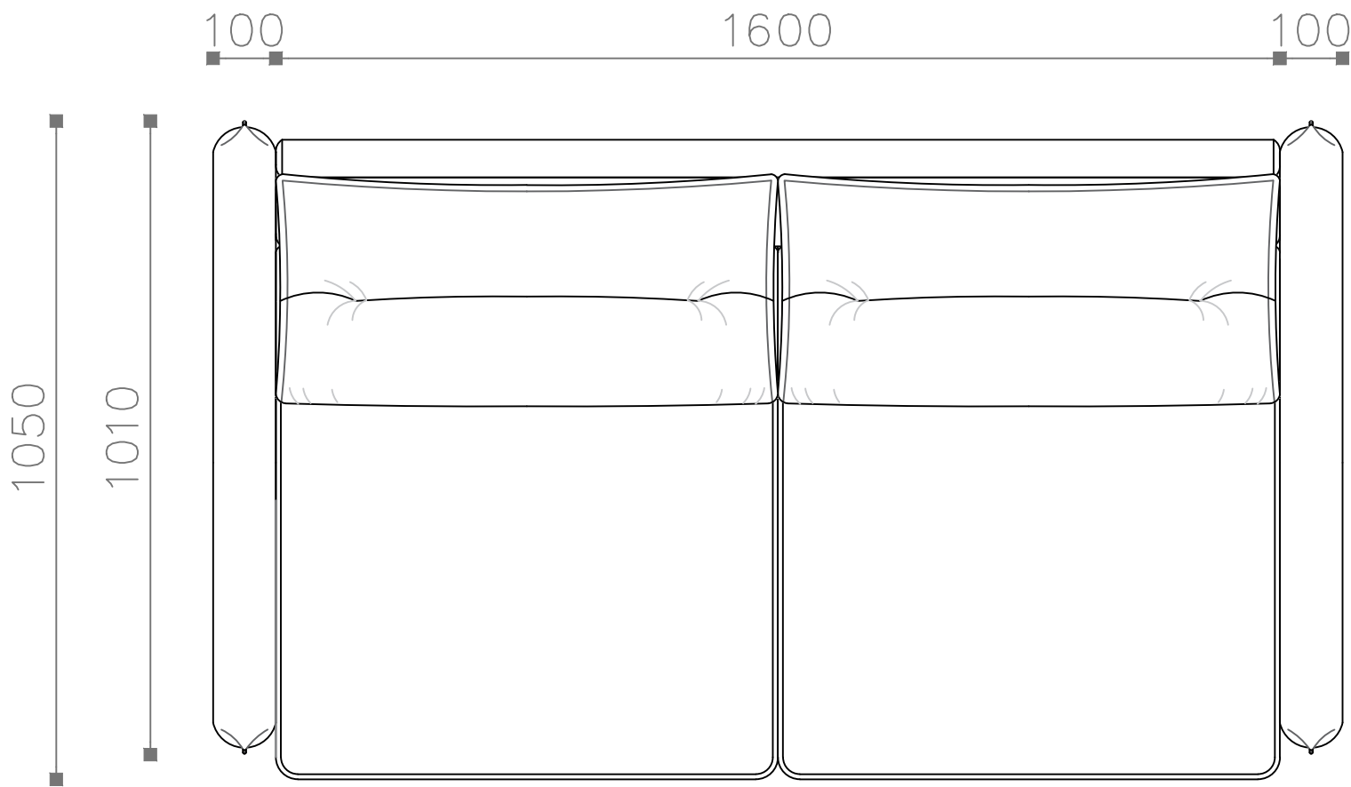
Диван-кровать 180 (ДКР 180) Вид сверху
