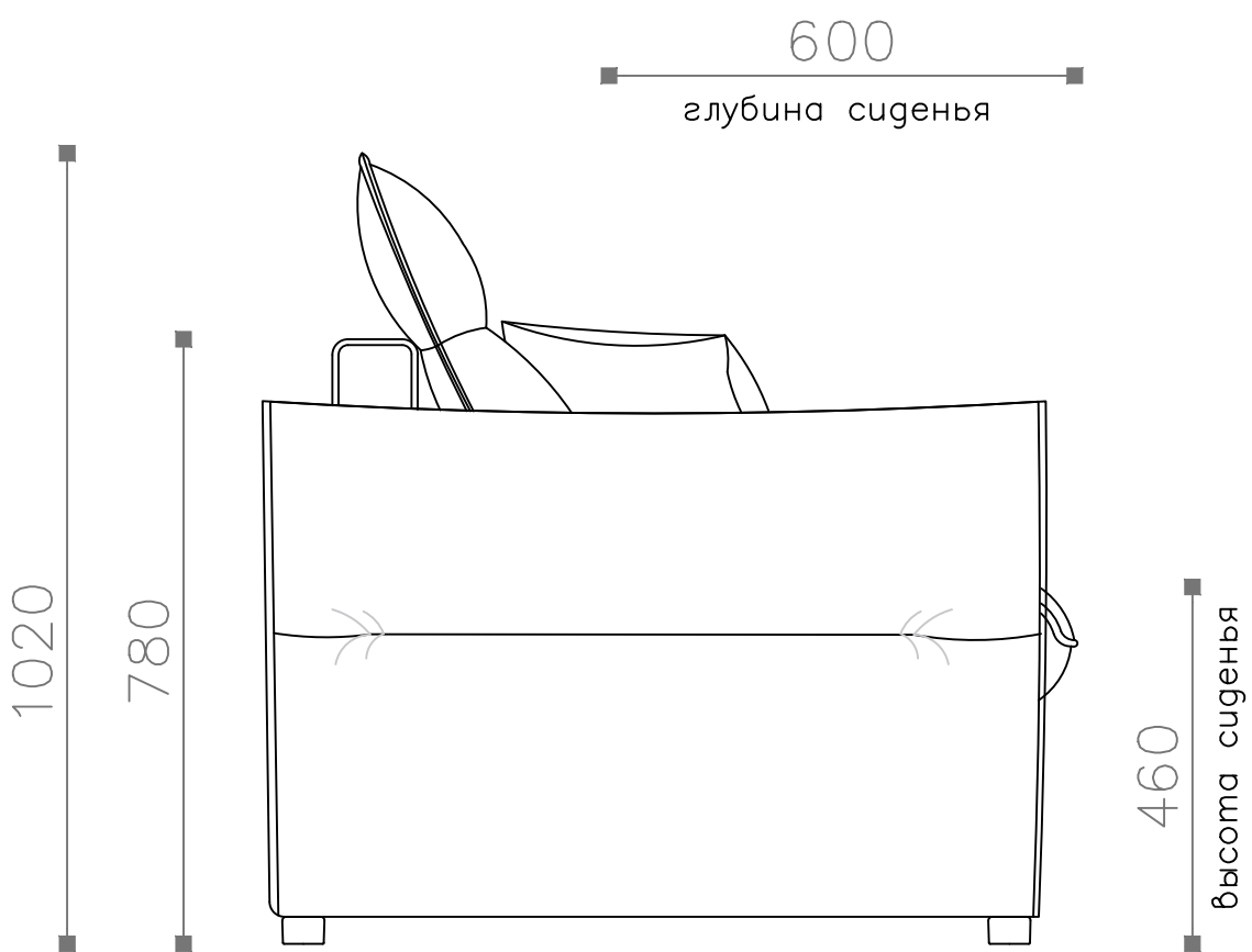
Диван-кровать 180 (ДКР 180) Вид сбоку
