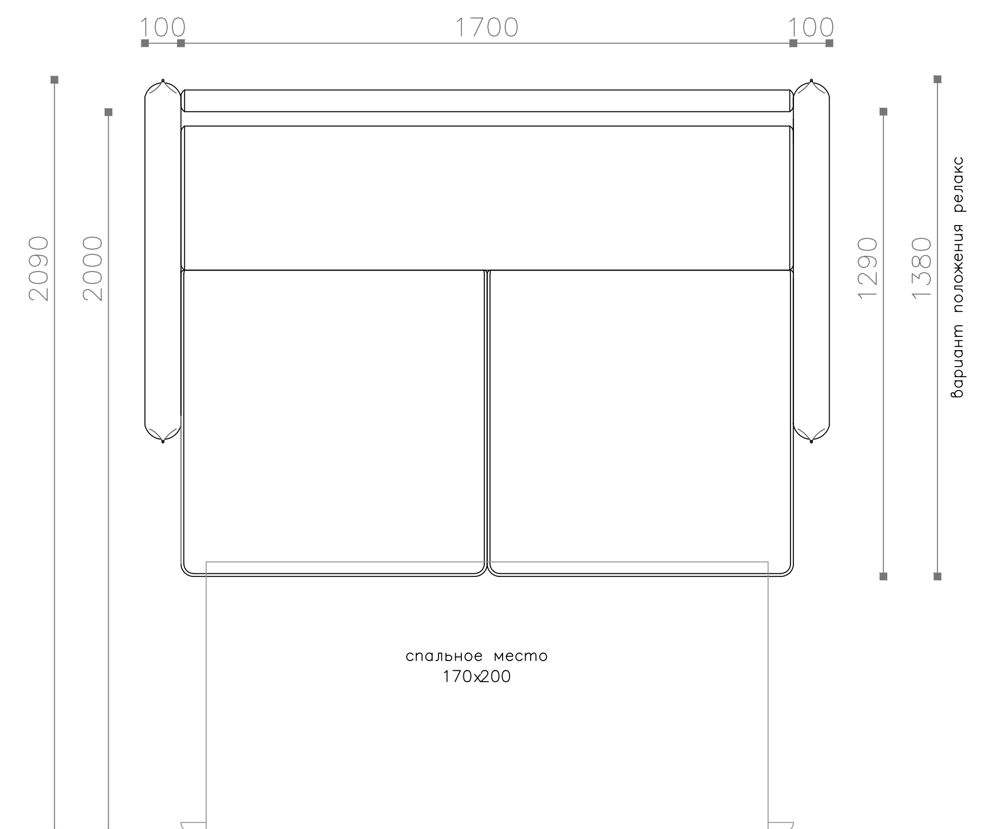
Диван-кровать 190 (ДКР 190) в разложенном виде Вид сверху
