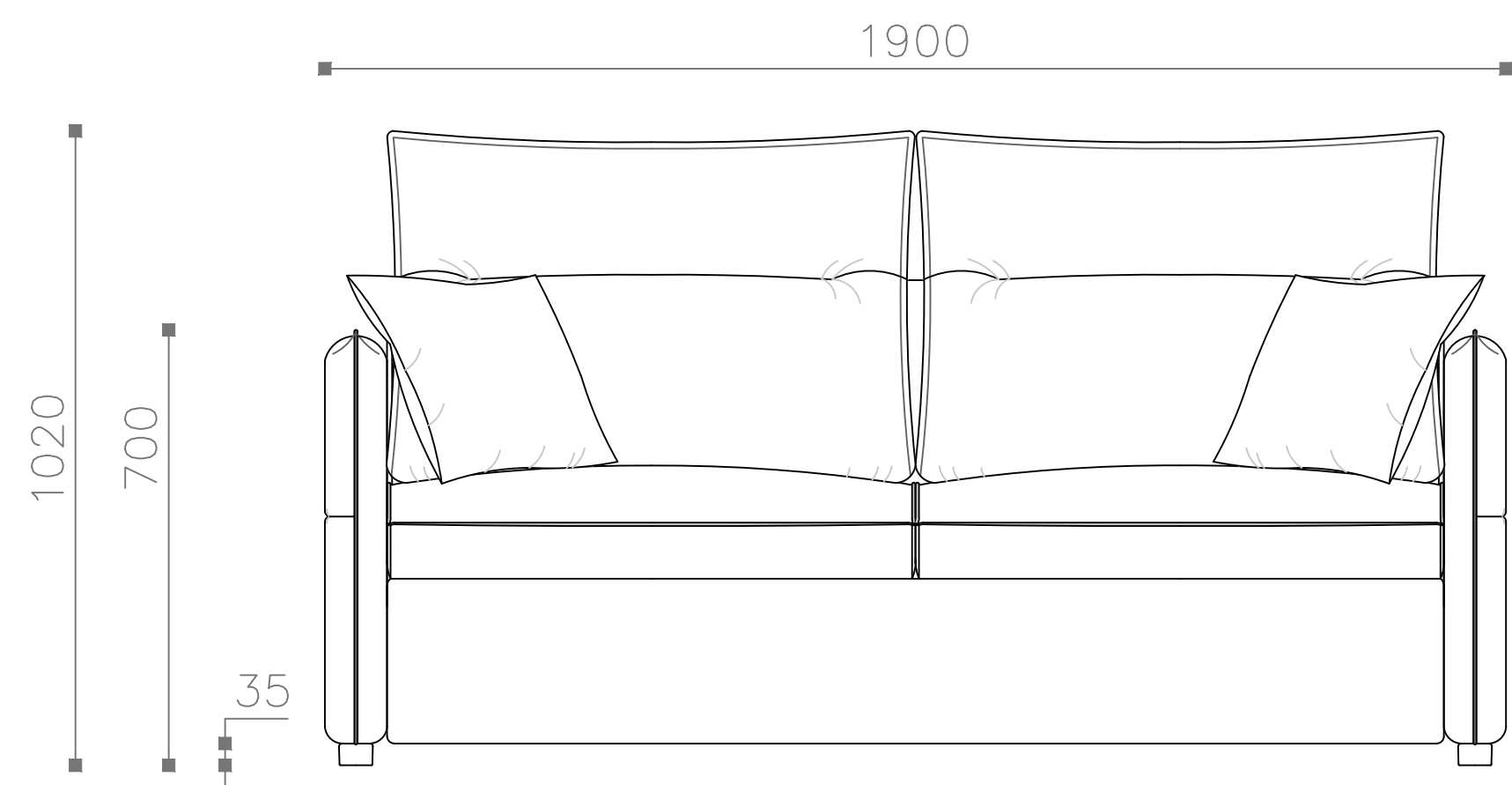
Диван-кровать 190 (ДКР 190) Фронтальный вид
