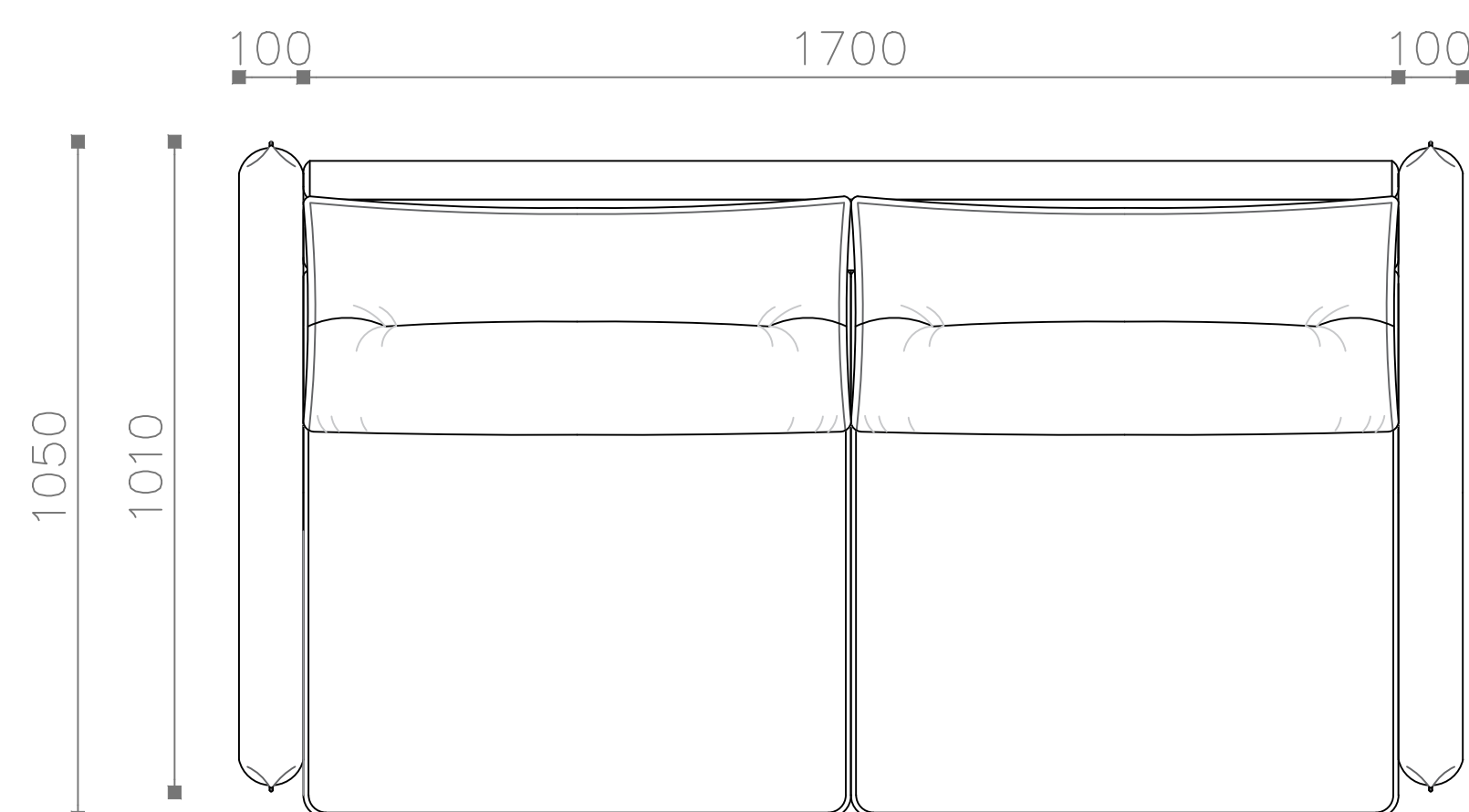
Диван-кровать 190 (ДКР 190) Вид сверху
