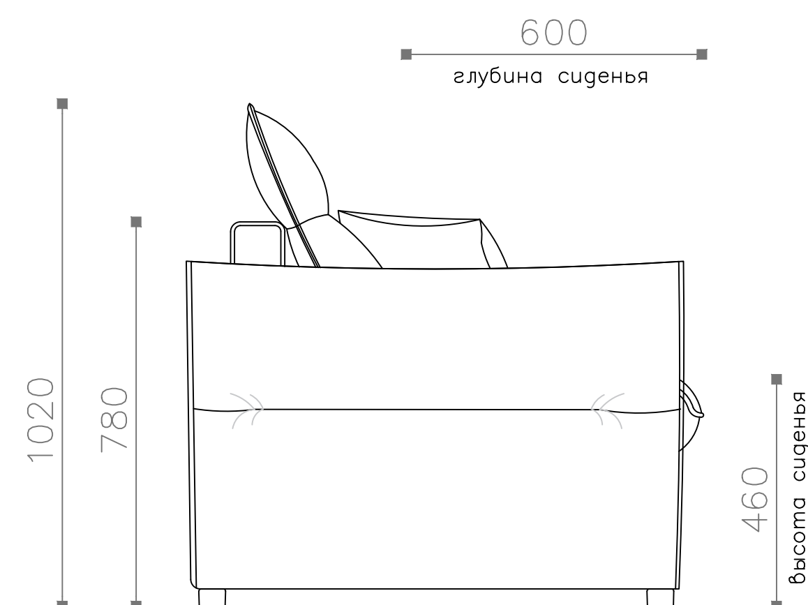
Диван-кровать 190 (ДКР 190) Вид сбоку
