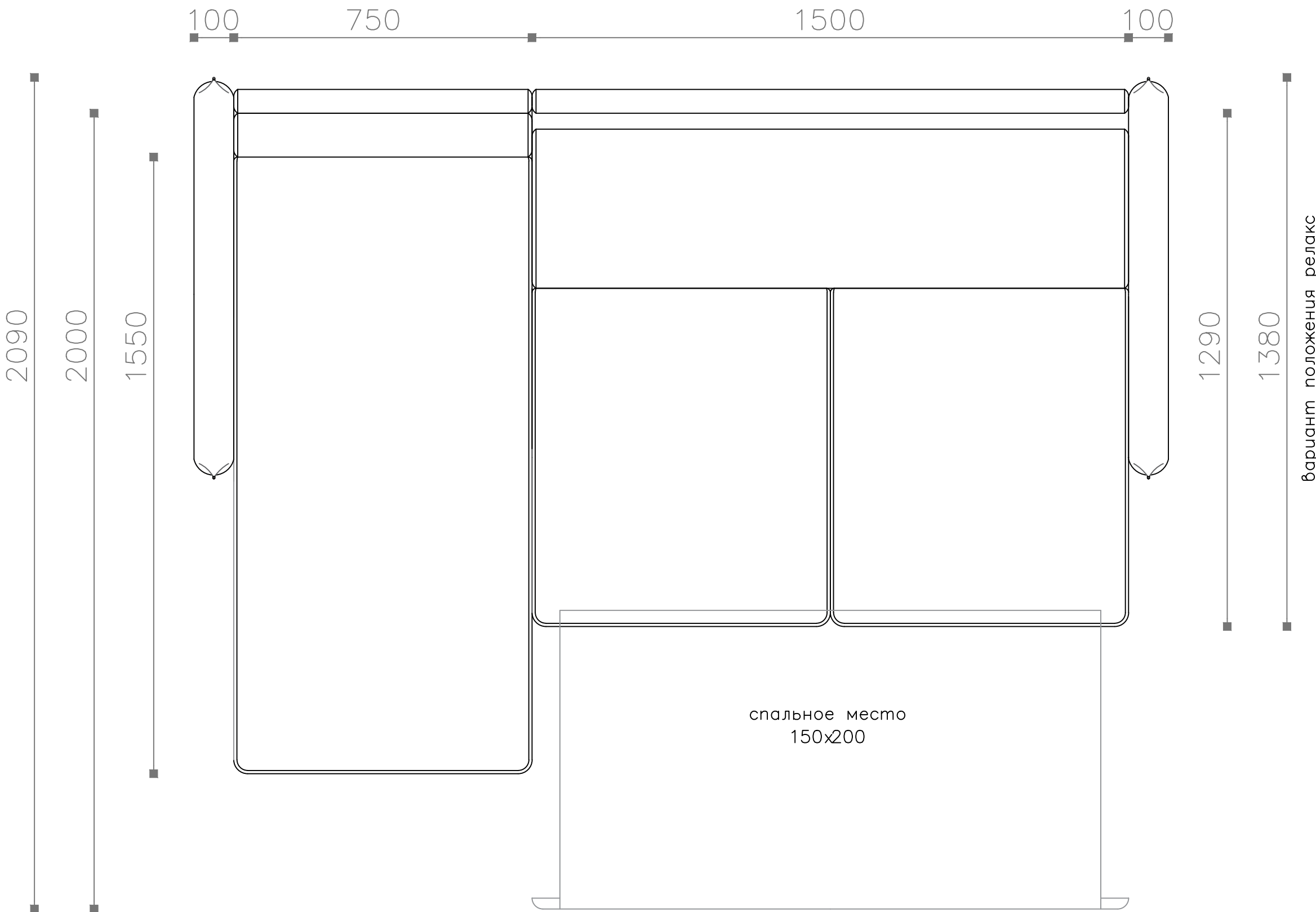
Угловой диван-кровать 245 (ДКУ 245) в разложенном виде Вид сверху
