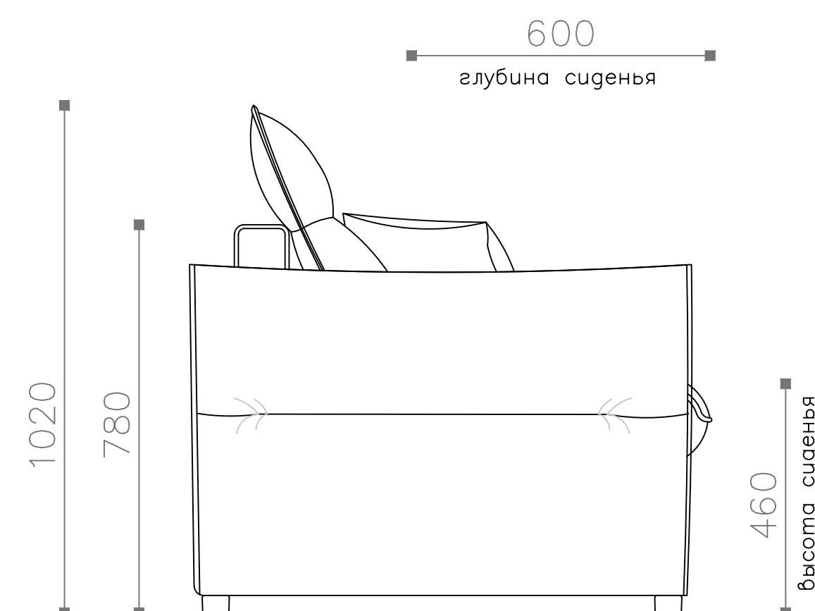
Кресло-кровать 100 (ККР 100) Вид сбоку
