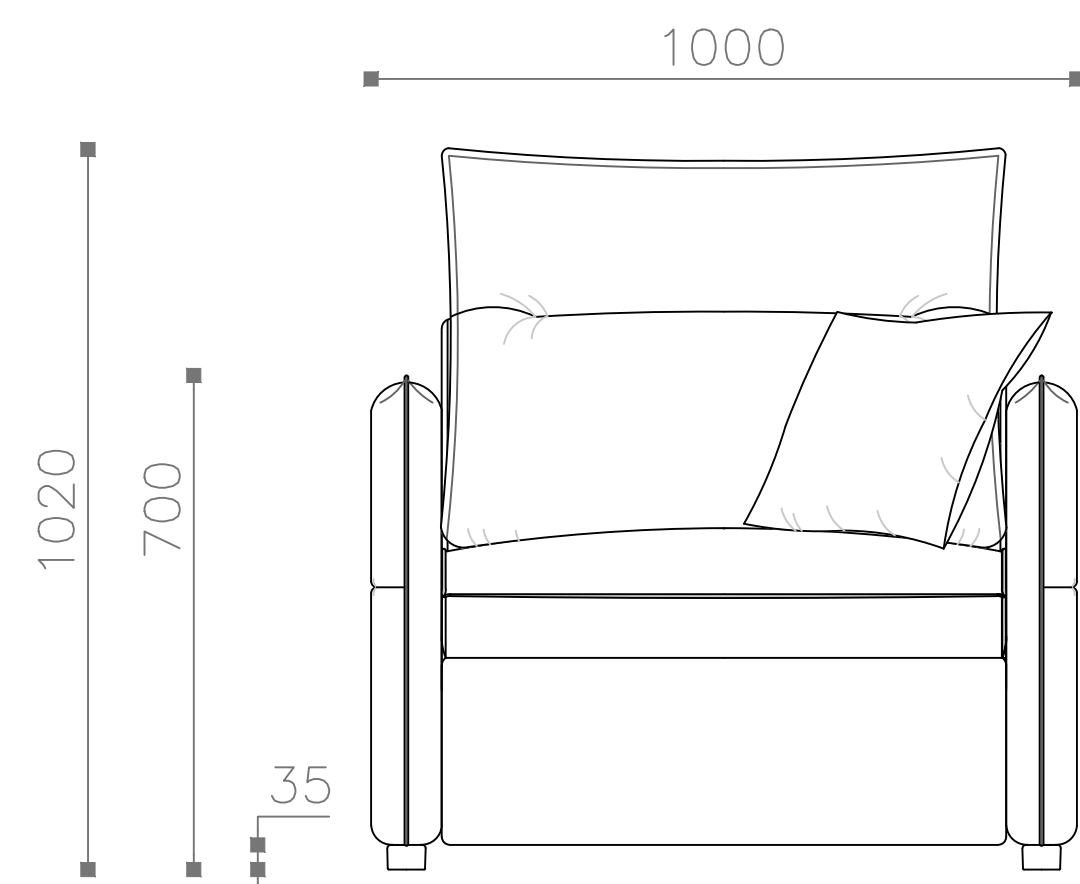
Кресло-кровать 100 (ККР 100) Фронтальный вид
