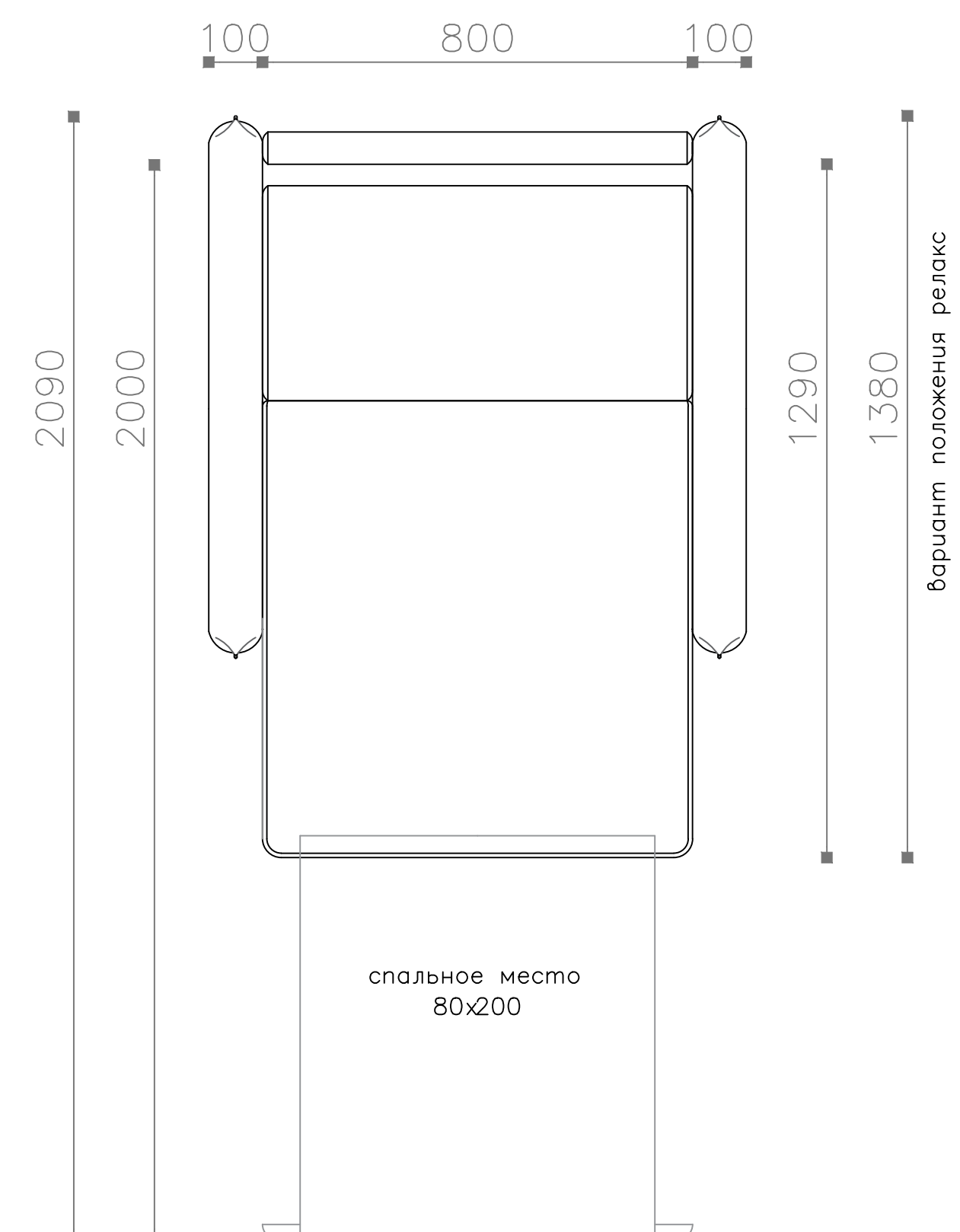
Кресло-кровать 100 (ККР 100) в разложенном виде Вид сверху
