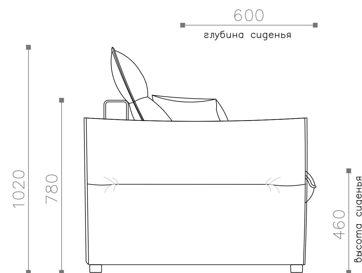
Кресло-кровать 105 (ККР 105) Вид сбоку
