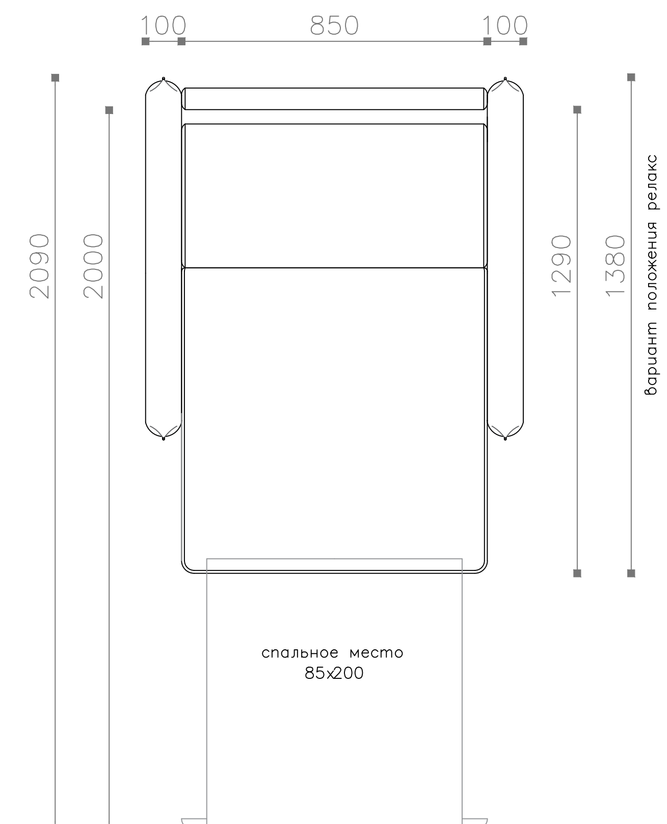
Кресло-кровать 105 (ККР 105) в разложенном виде Вид сверху
