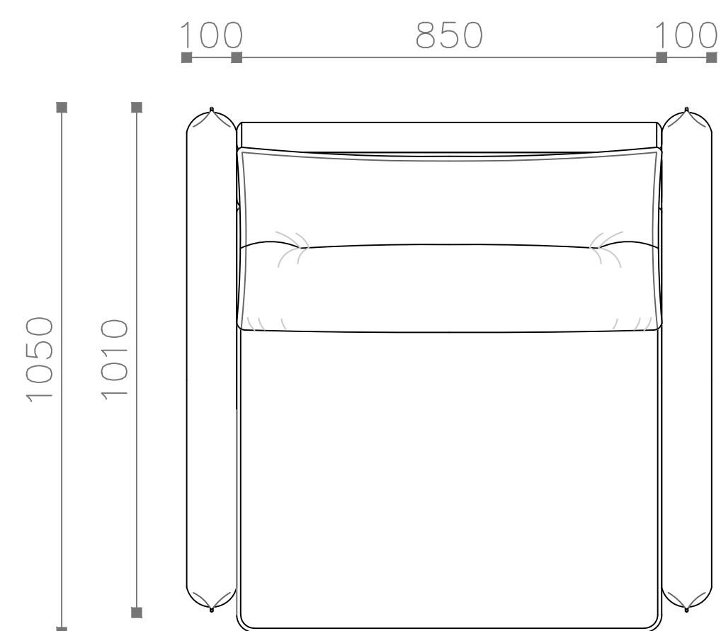
Кресло-кровать 105 (ККР 105) Вид сверху
