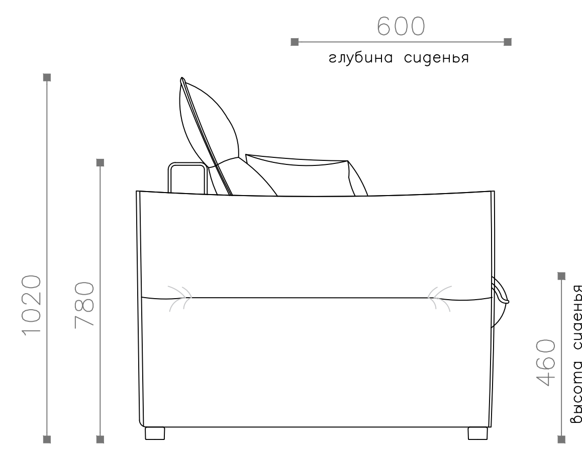
Кресло-кровать 90 (ККР 90) Вид сбоку
