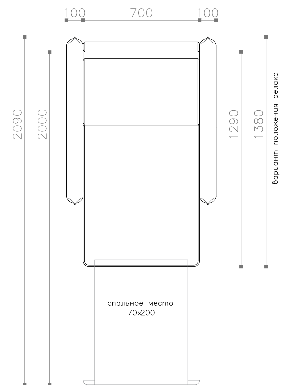
Кресло-кровать 90 (ККР 90) в разложенном виде Вид сверху
