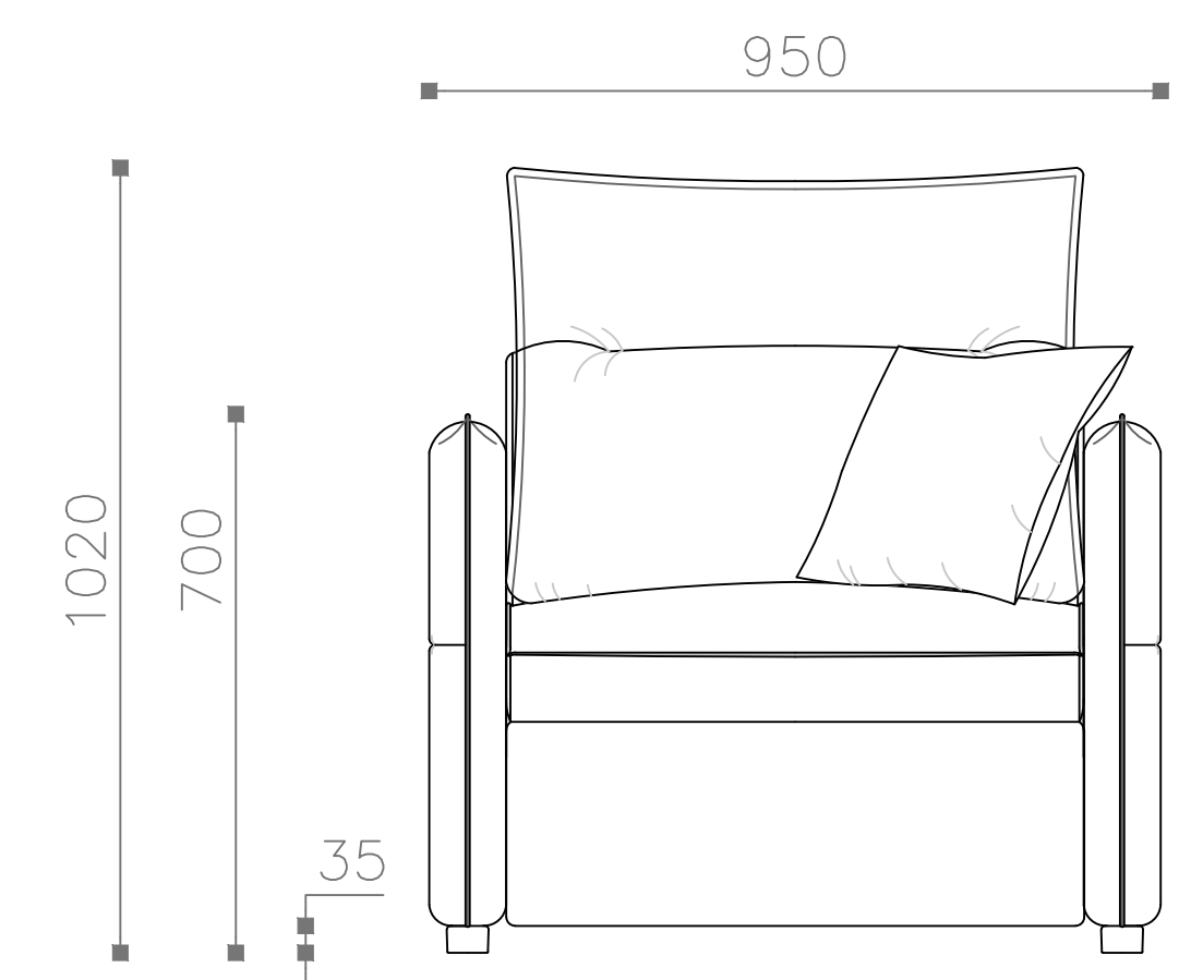
Кресло-кровать 95 (ККР 95) Фронтальный вид
