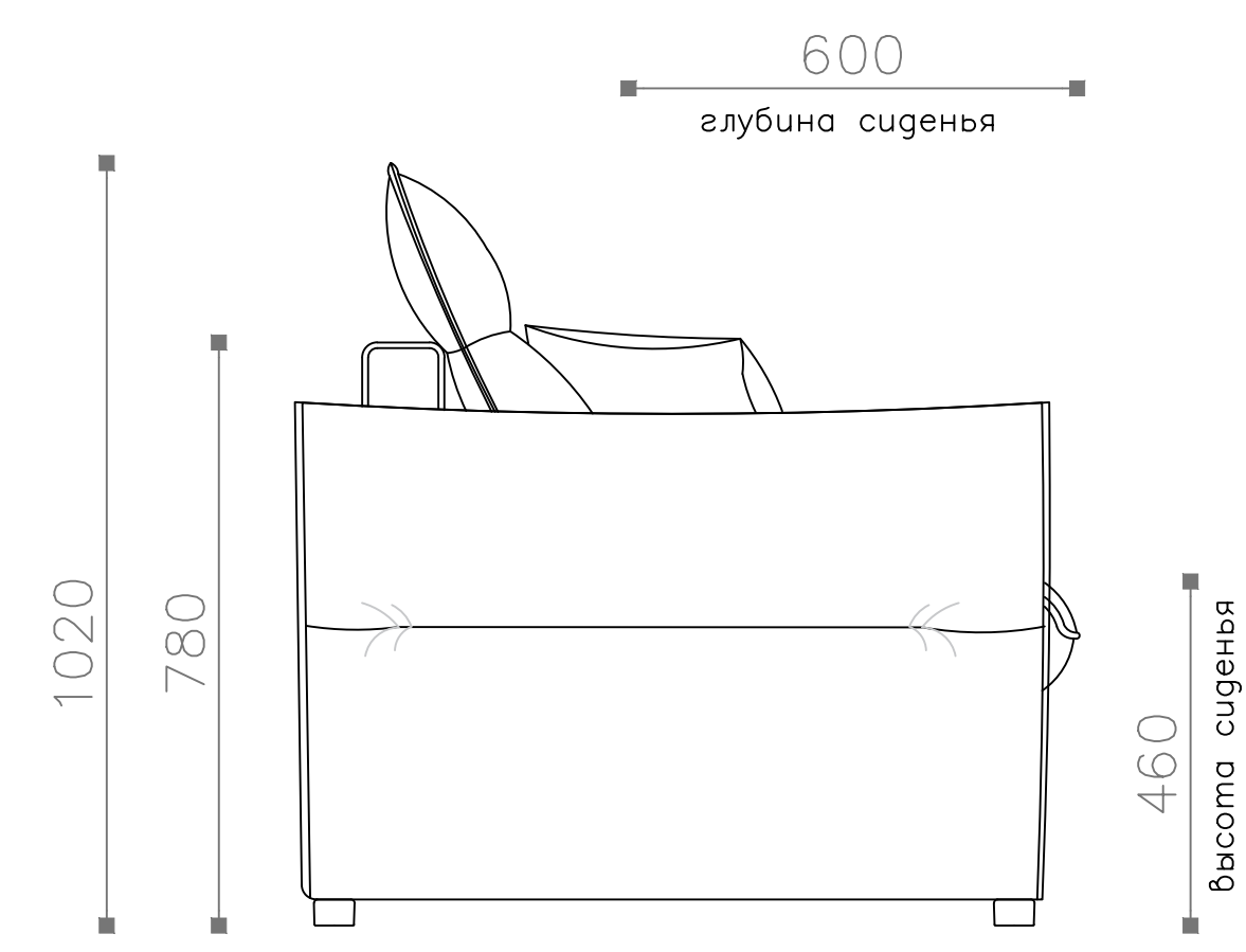
Кресло-кровать 95 (ККР 95) Вид сбоку
