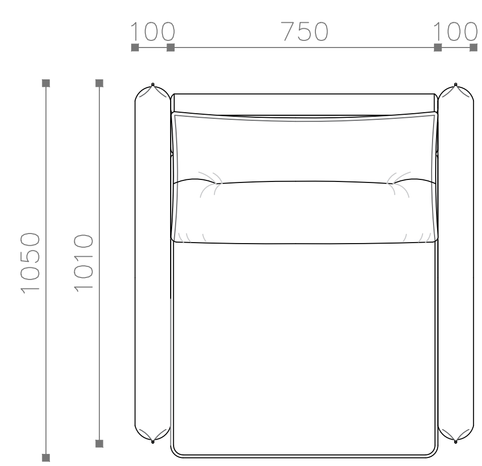
Кресло-кровать 95 (ККР 95) Вид сверху
