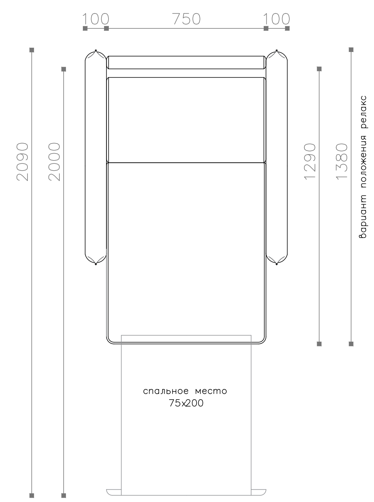
Кресло-кровать 95 (ККР 95) в разложенном виде Вид сверху
