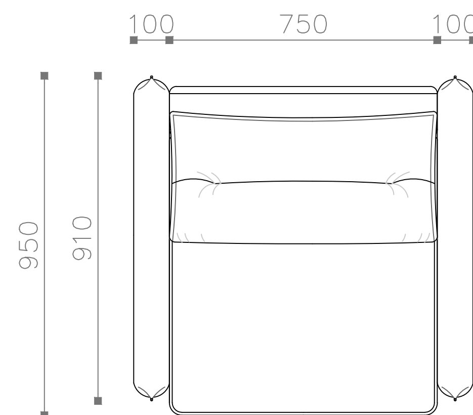
Кресло-кровать 95 (ККР 95) Вид сверху
