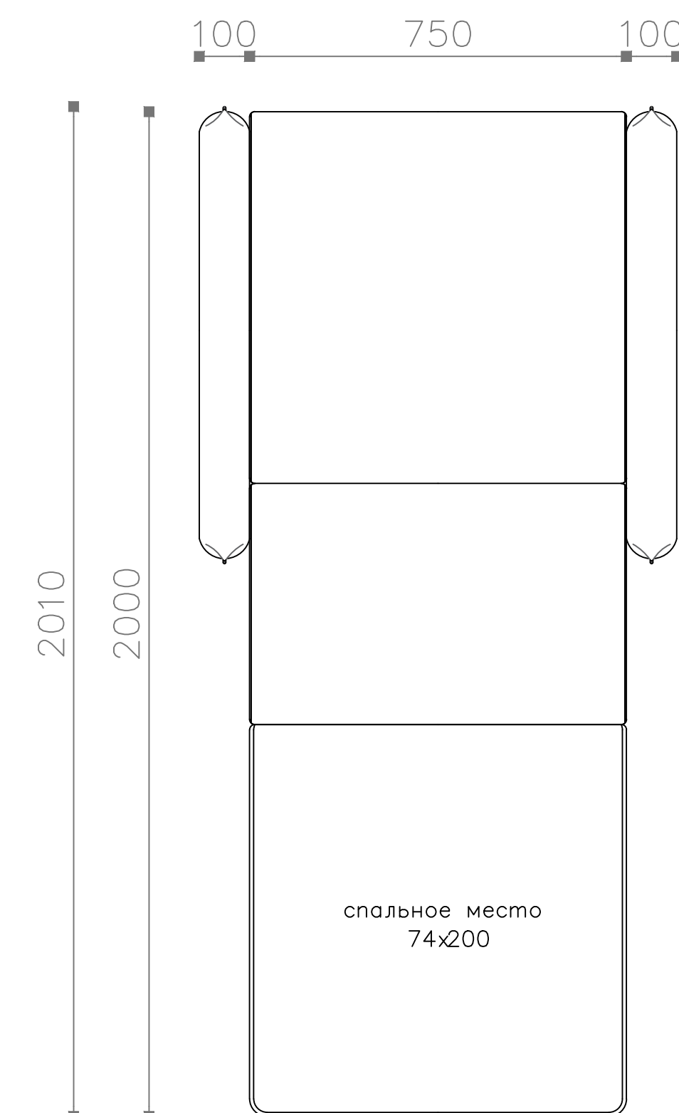
Кресло-кровать 95 (ККР 95) в разложенном виде Вид сверху
