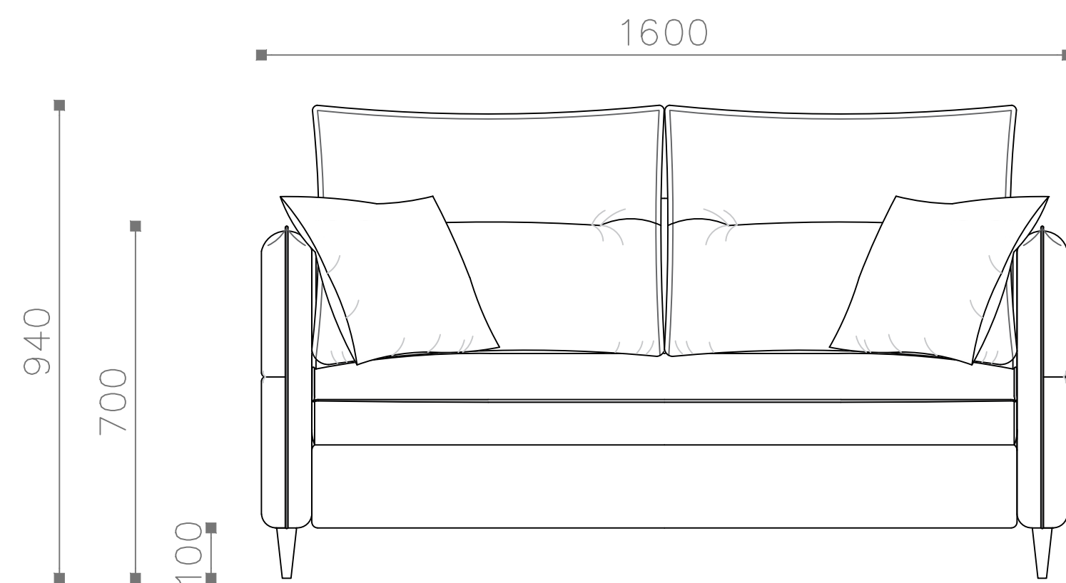
Диван-кровать 160 (ДКР 160) Фронтальный вид
