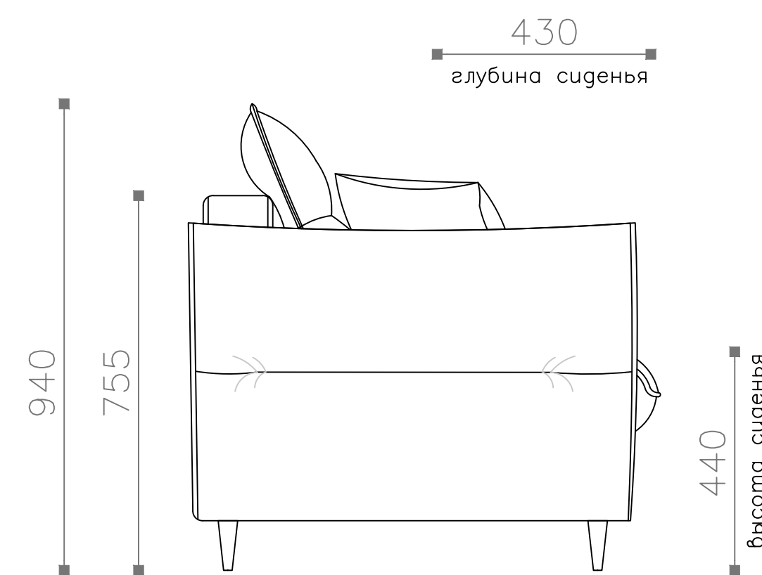
Диван-кровать 160 (ДКР 160) Вид сбоку
