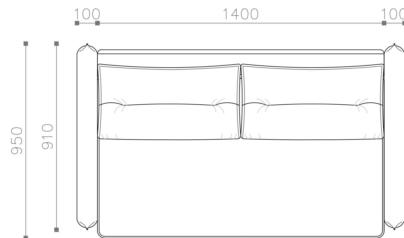
Диван-кровать 160 (ДКР 160) Вид сверху
